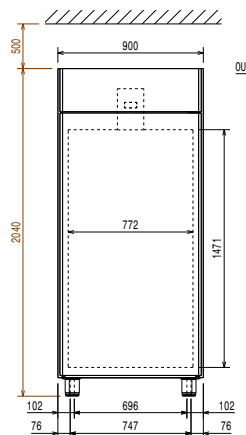
Front aanzicht
