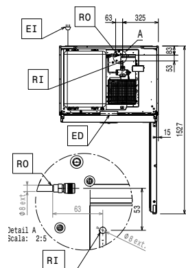
Boven aanzicht
